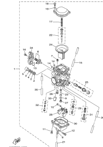
FIG. 8 CARBURADOR
