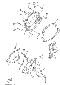
FIG. 11 TAMPA DA CARÇAÇA
