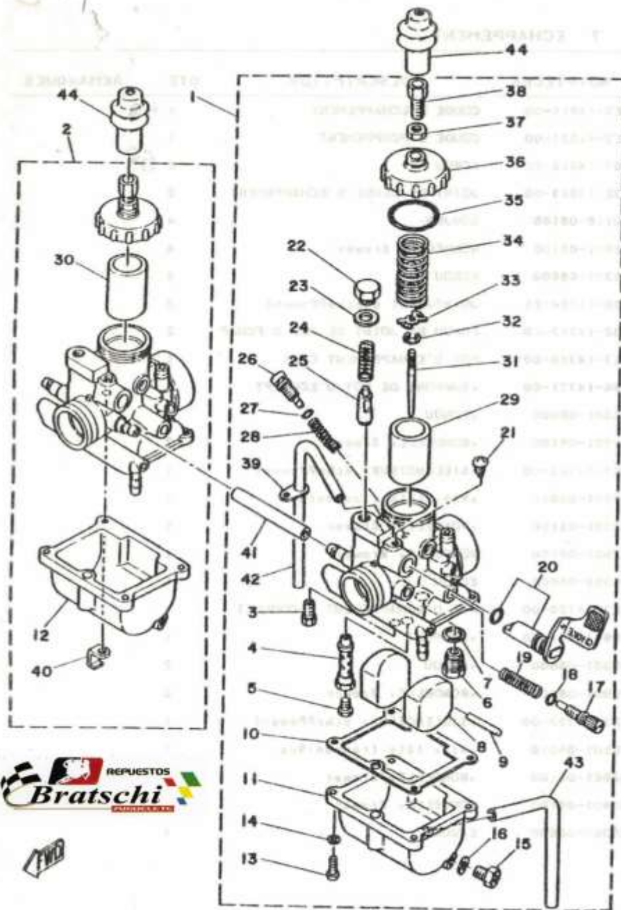
FIG. 6 CARBURATEUR
