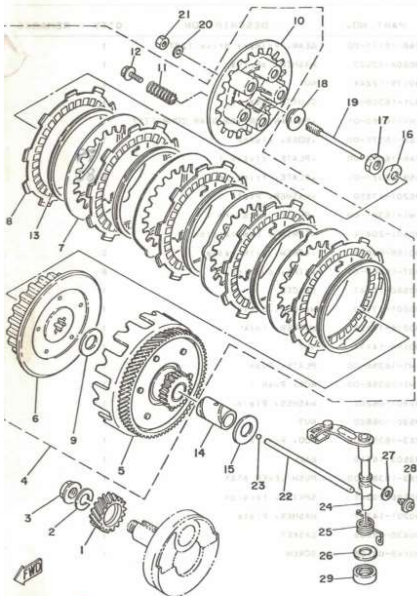
FIG. 11 CLUTCH
