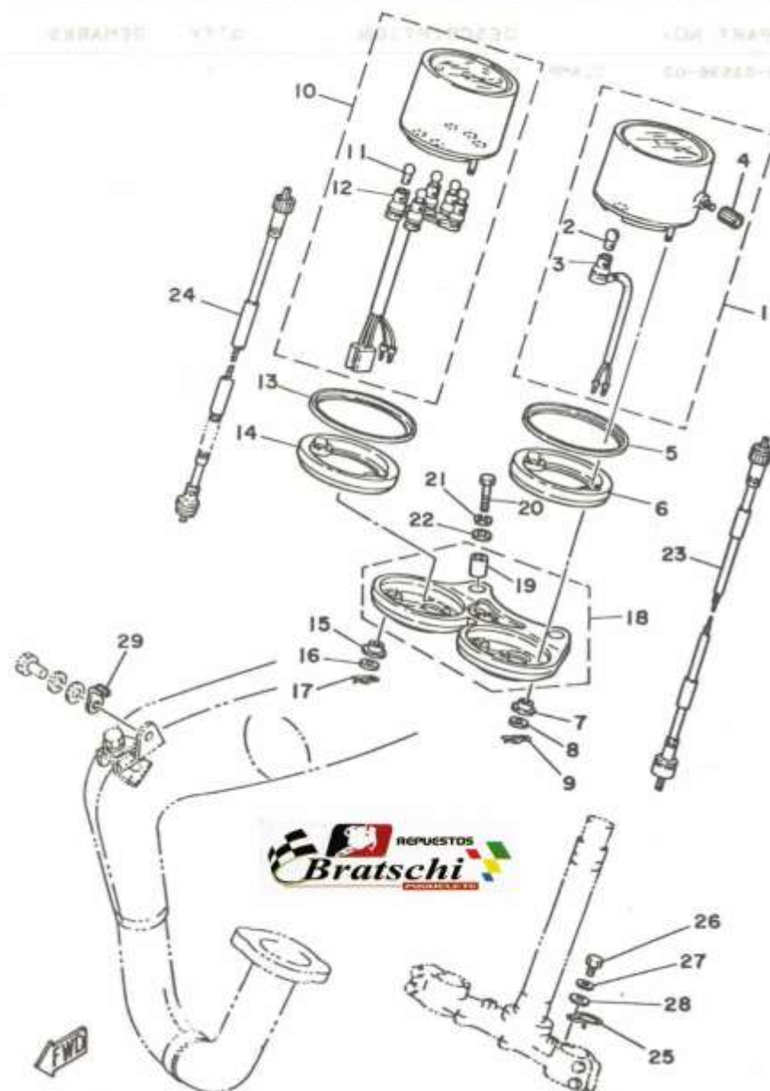
FIG. 31 METER
