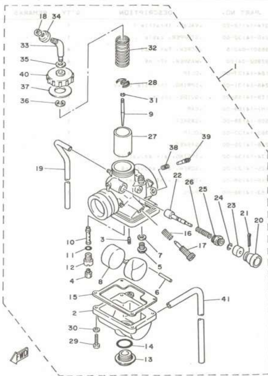
FIG. 6 CARBURETOR
