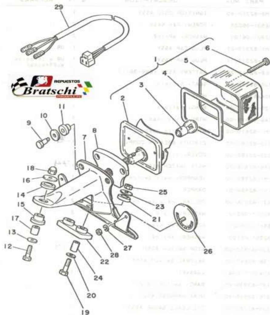
FIG. 33 TAILLIGHT
