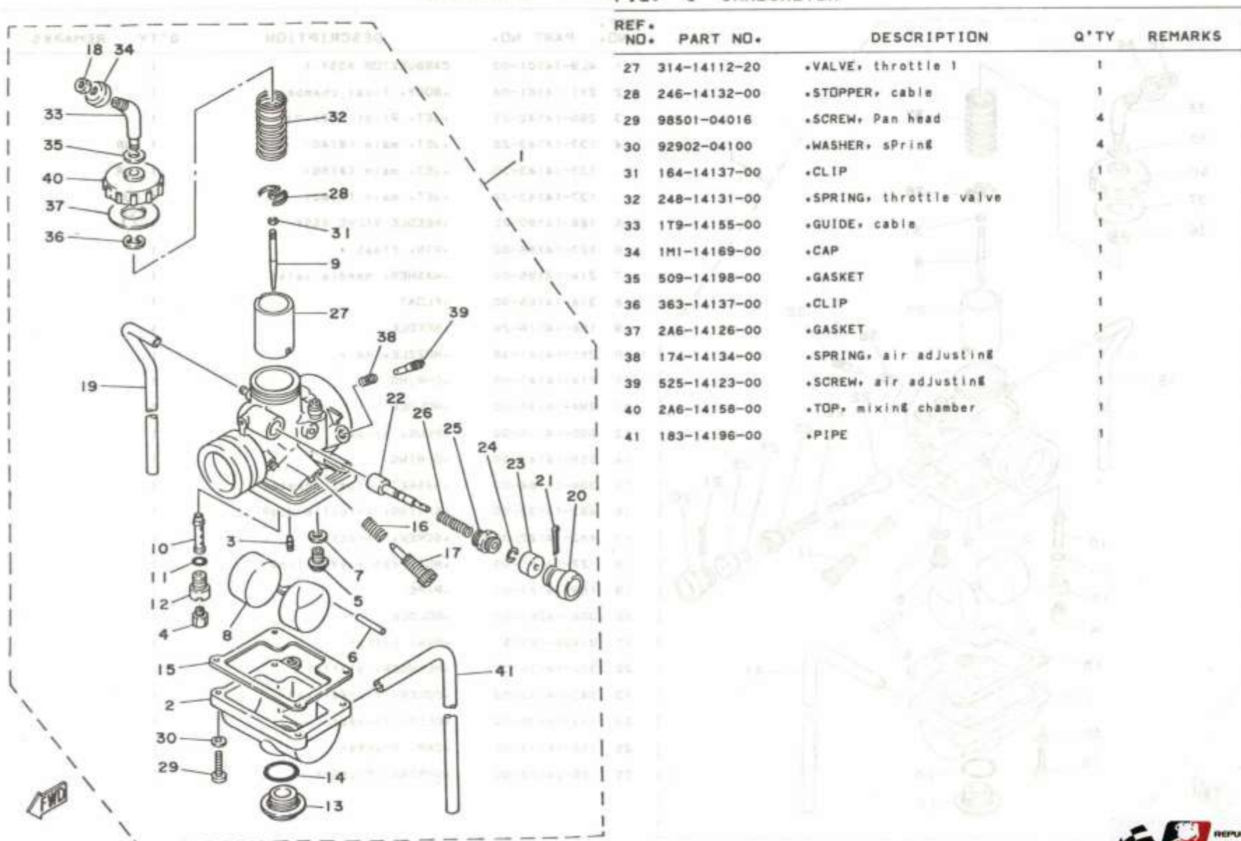
FIG. 6 CARBURETOR
