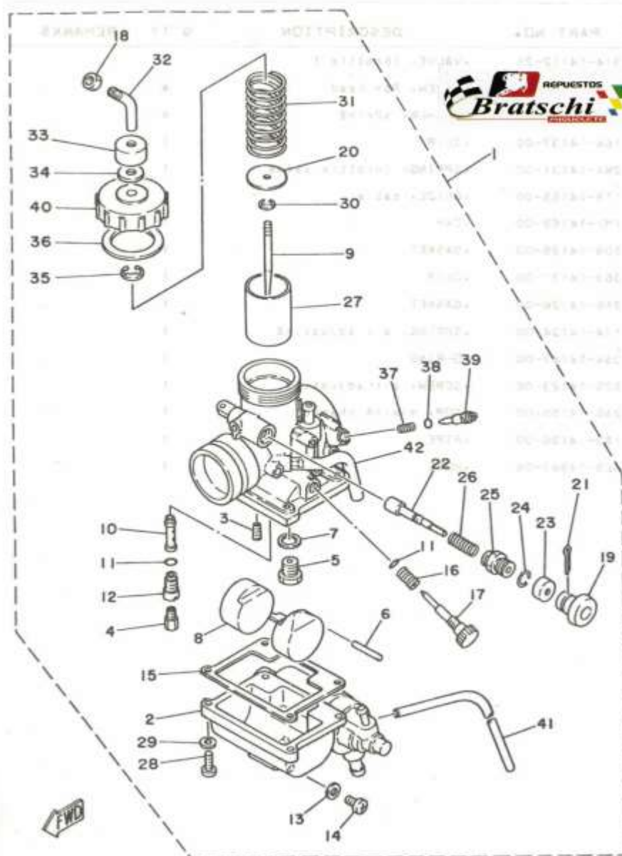
FIG. 39 CARBURETOR
