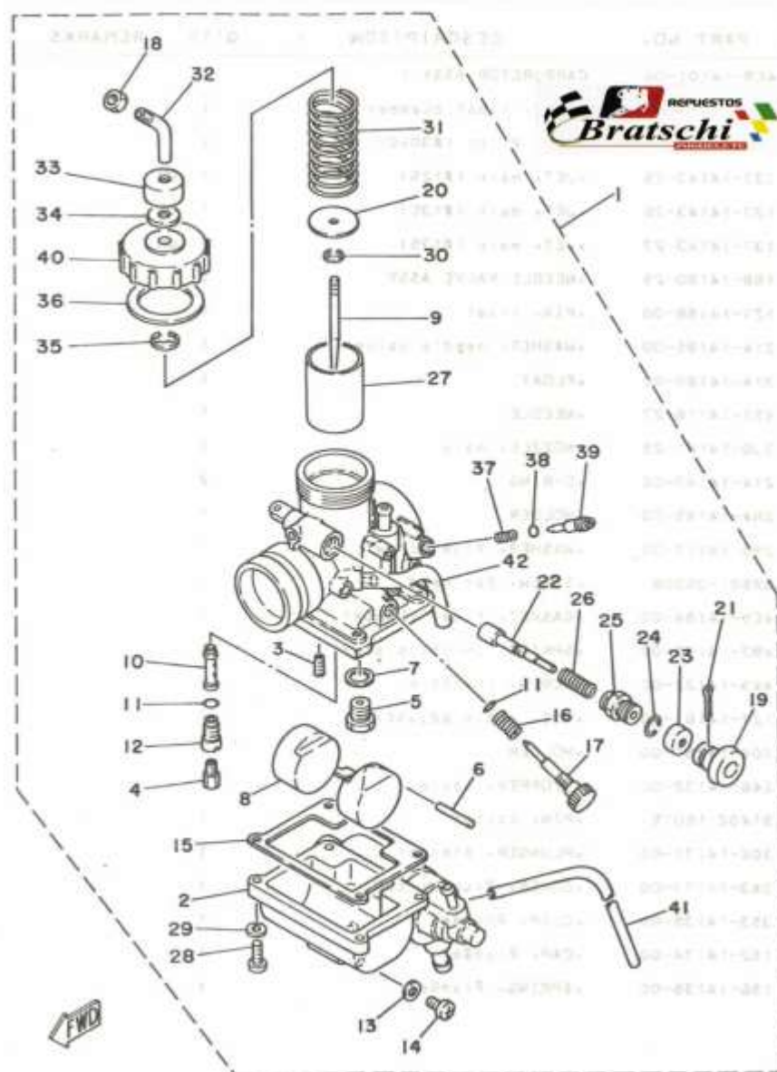
FIG. 39 CARBURETOR
