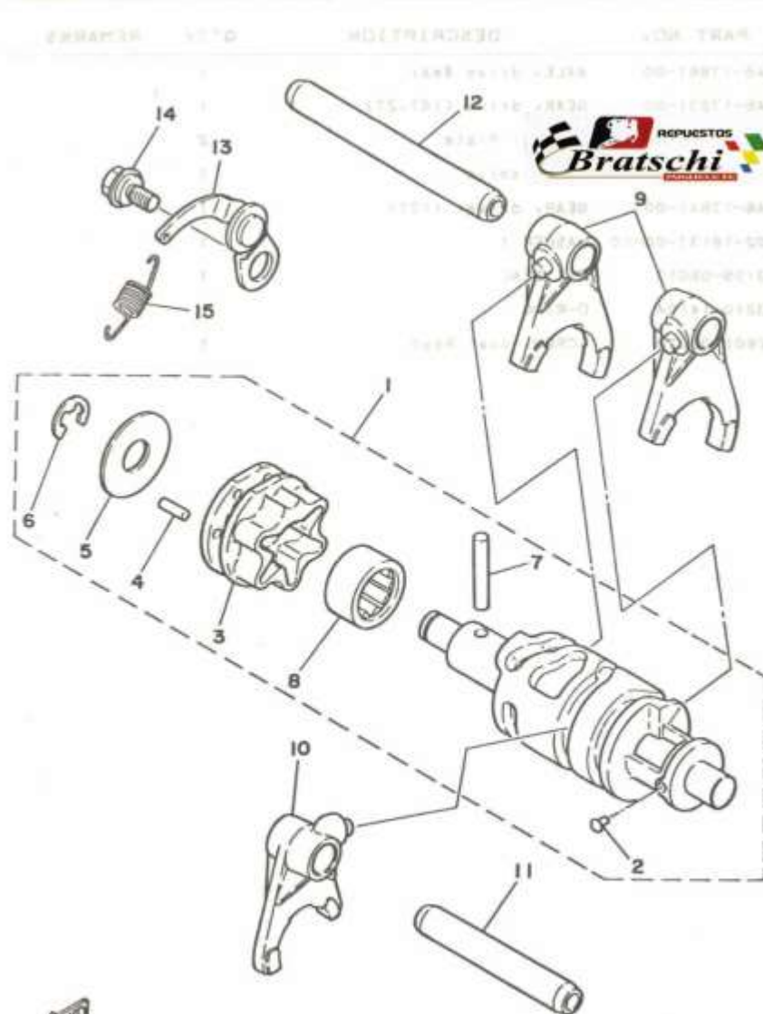
FIG. 14 SHIFT CAM-FORK
