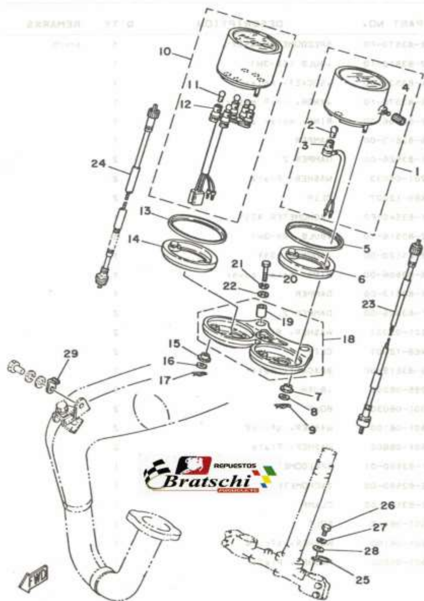
FIG. 31 METER
