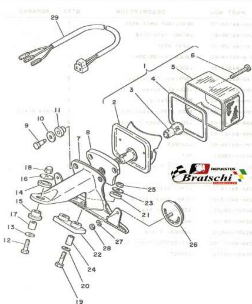
FIG. 33 TAILLIGHT
