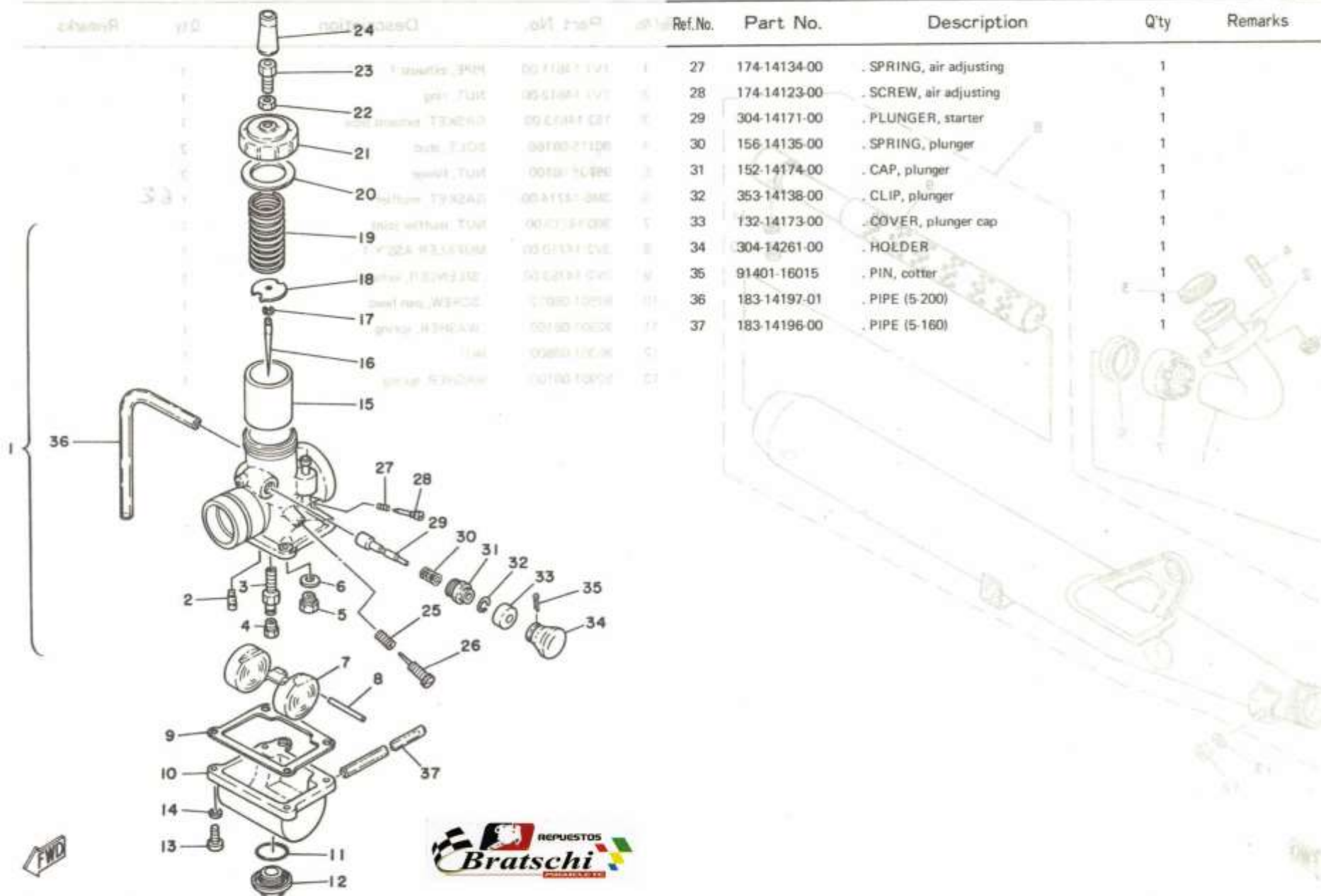
Fig. 6 Carburetor
